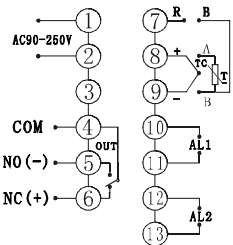
CD800接线图
