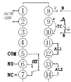
CD700接线图
