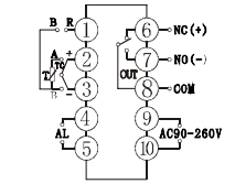
CD100只有一路报警输出(AL2)
