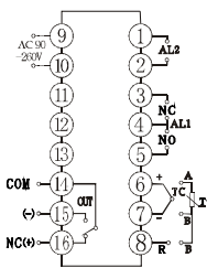
CD400-500接线图
