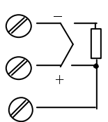
仪表对应接线图
